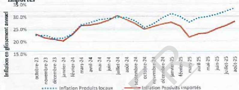
Graphique 9: Inflation en glissement annuel des produits locaux et importés
