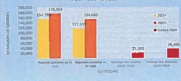
Graphique 11 Recettes, dépenses, et variations cumulées au 31 Août 2024 & 2025
