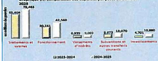
Graphique 14: comparaison des dépenses par poste au 31 Août
