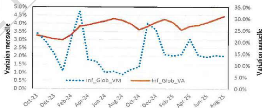
Graphique 8: Inflation globale en variation mensuelle et annuelle
