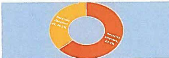
Graphique 12: Répartition des recettes selon leur origine et leur contribution relative- Au 31 Août 2025
